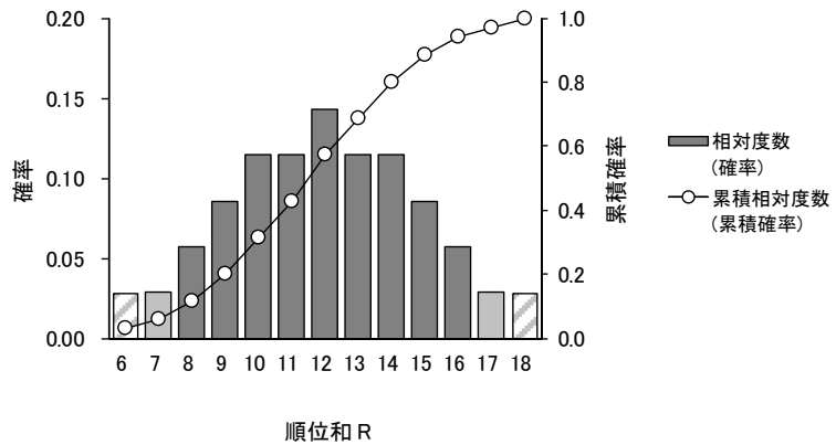
図-2. n_1=3, n_2=4 の場合の順位和の確率分布
